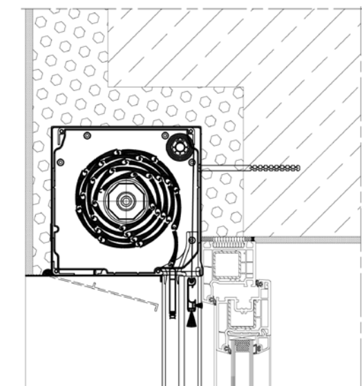
SP-E - Rollläden
