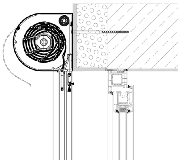
SKO - Rollläden
