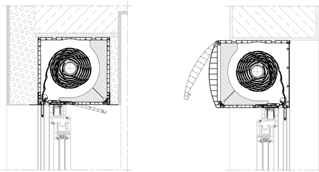
SKT - Rollläden
