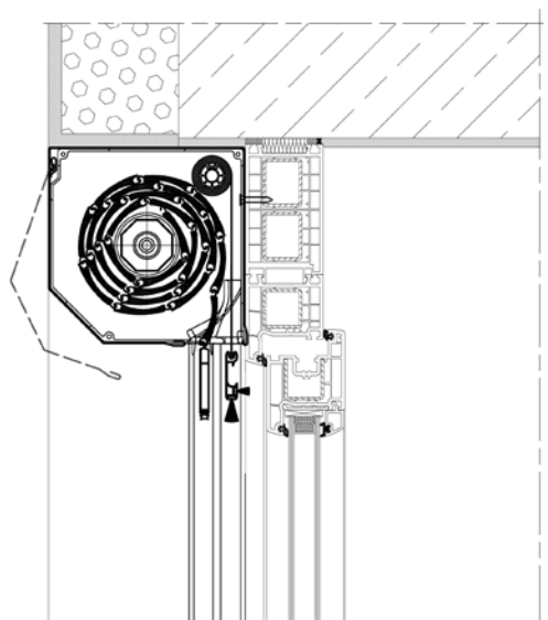
SK – Rollläden
