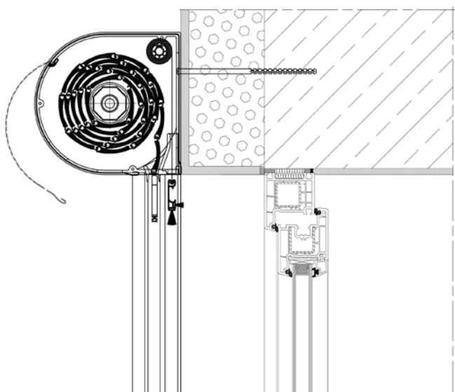
SKO-P - Rollläden
