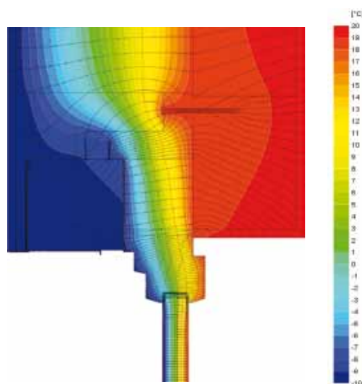
Verteilung der Isothermen
