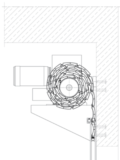
Tor – BPR/KNS
