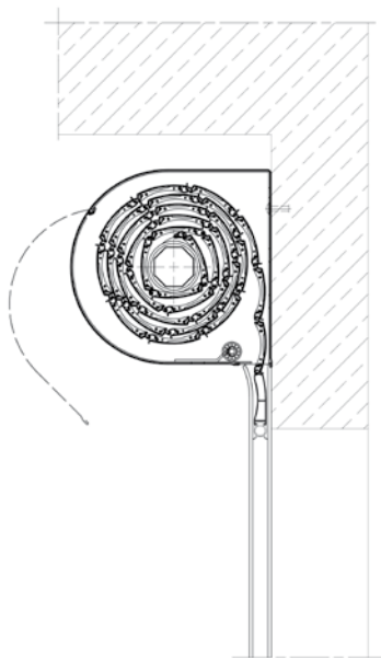
Gitter – BKR/SKO-P
