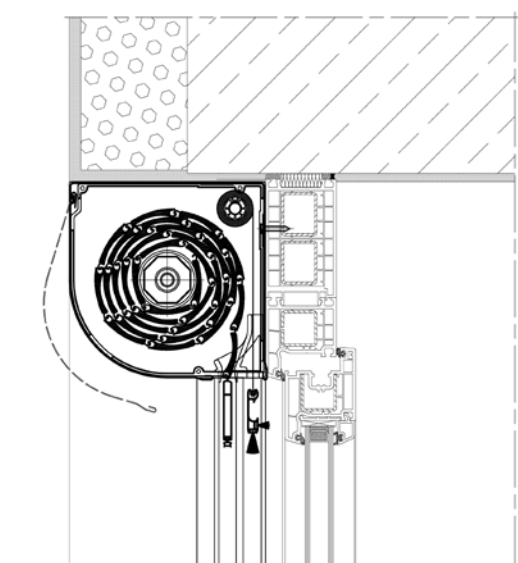
SKP – Rollläden
